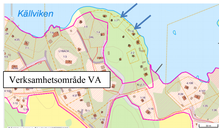
Figur 1. Aktuella fastigheter Augustendal 1:6 och 1:7 (markerade med pilar) samt nuvarande verksamhetsområde för allmän VA-anläggning i Eskilstuna kommun. Det allmänna VA-ledningsstråket är markerat med röd linje.
