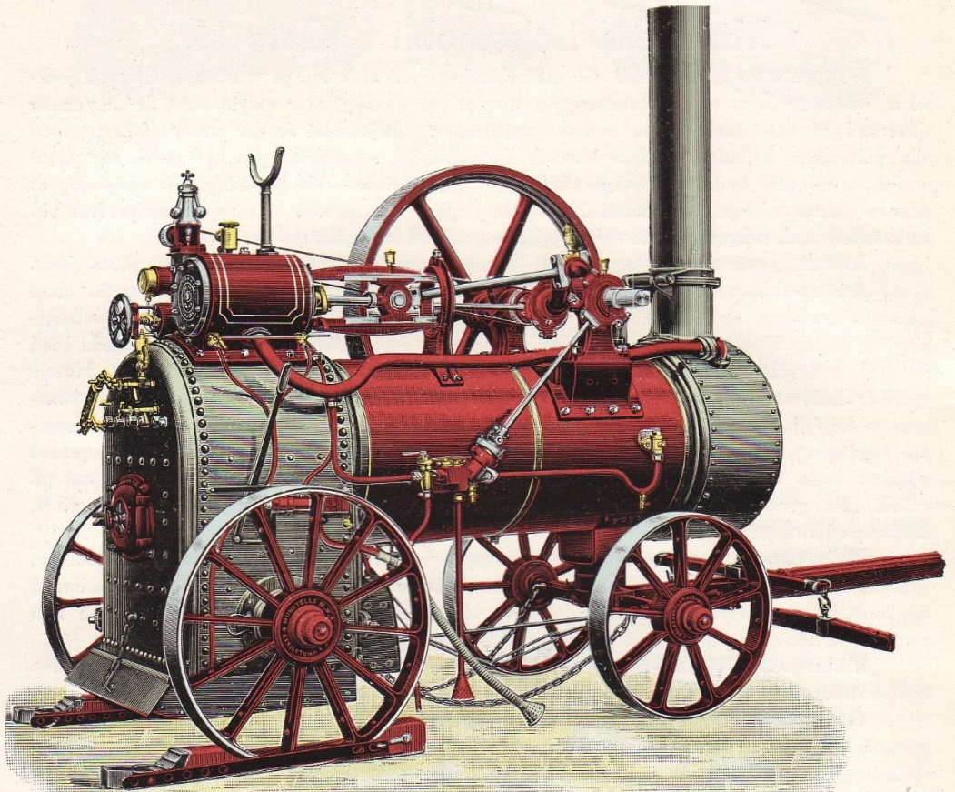
Munktells enkelcylindriga Lokomobil. Klass H.
